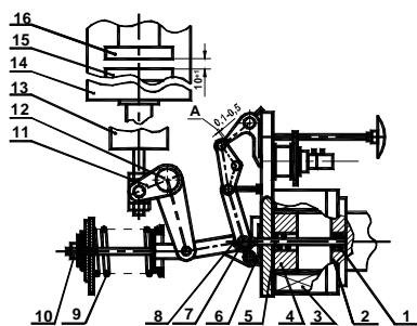
Выключатель отключен Рис.3а
