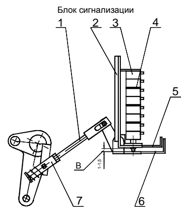
(включенное положение выключателя)
