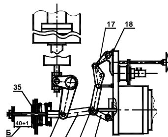
Выключатель включен Рис.3б
