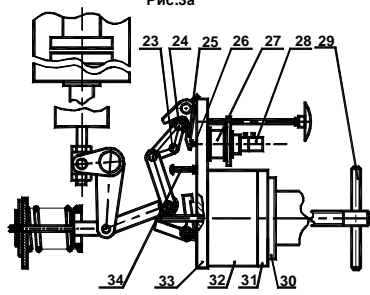
Промежуточное положение выключателя Рис.3в
